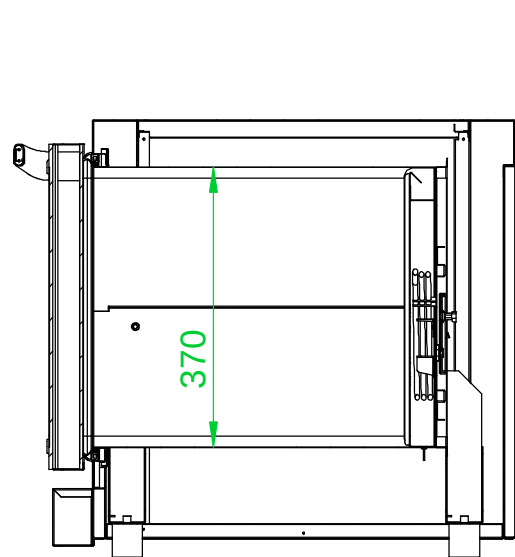
SEZIONE B-B
